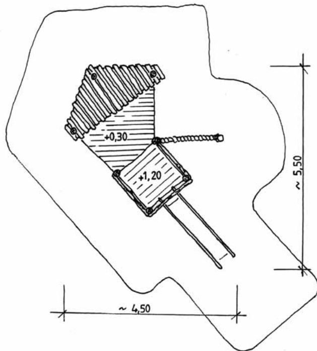
Pantoffel-Kombination 085105R
