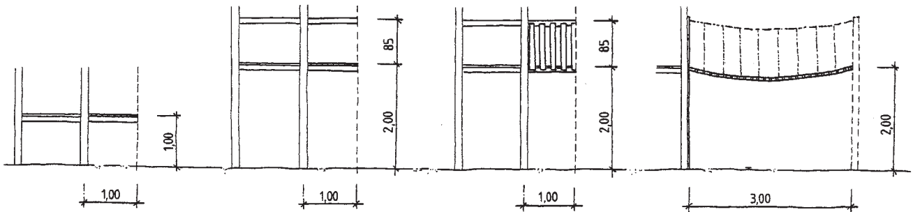
SCHRÄGES KLETTERNETZ 08 4058 SCHRÄGES KLETTERNETZ 08 4059 SCHRÄGES KLETTERNETZ-TRAPEZ 08 4060 SCHRÄGES KLETTERNETZ 08 4068 SCHRÄGER REIFENAUFSTIEG 08 4061 KLETTERWAND 08 4098
