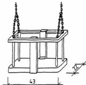
SICHERHEITS-SCHAUKELSTZ 02 0386
