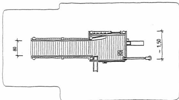
SANDSPIELHOF MIT BRÜCKE 092850 D
