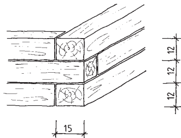
SANDKASTENEINFASSUNG 09 2705/1
