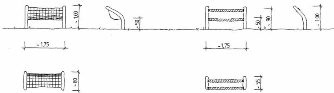
Netz - Sitz GAT 02 1500
