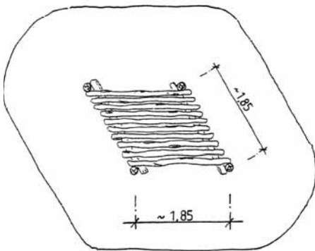
Stangensitz GAT 02 1601 R
