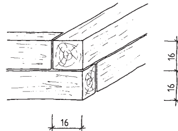
SANDKASTENEINFASSUNG 09 2705/2
