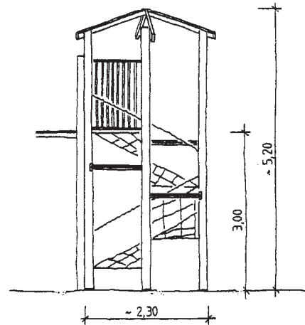
TAMPENBRÜCKE MIT 2 HANDSEILEN ØB 4084
