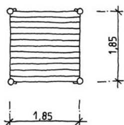
Viereck-Podest GAT 00 5019R
